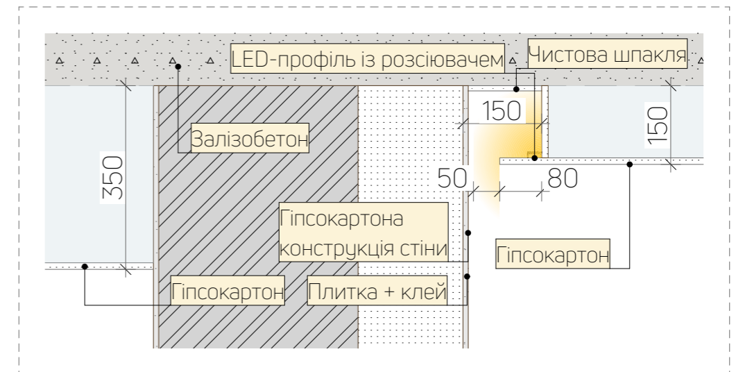
РОЗРІЗ 4-4
