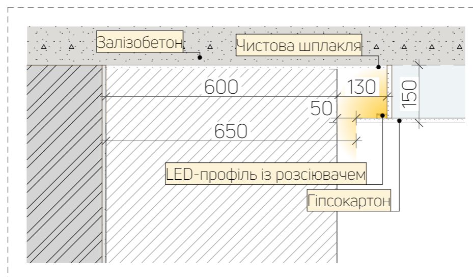
РОЗРІЗ 6-6
