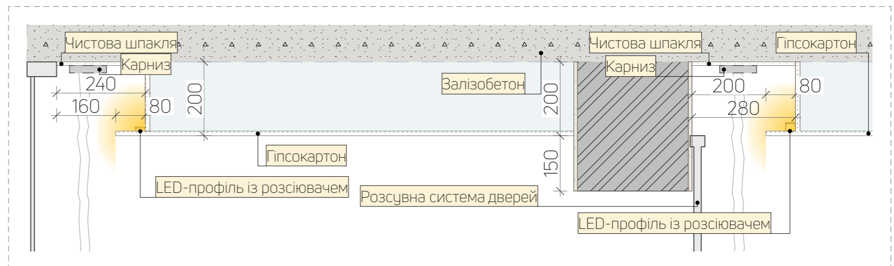
РОЗРІЗ 6-6
