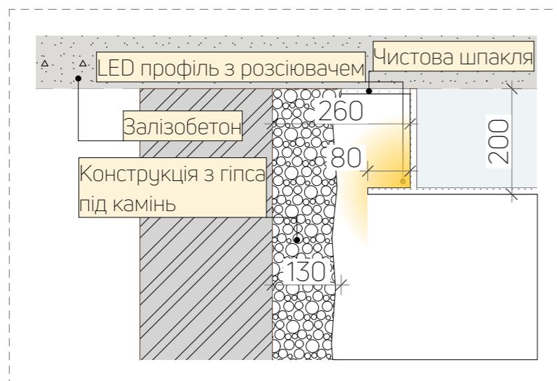
РОЗРІЗ 5-5
