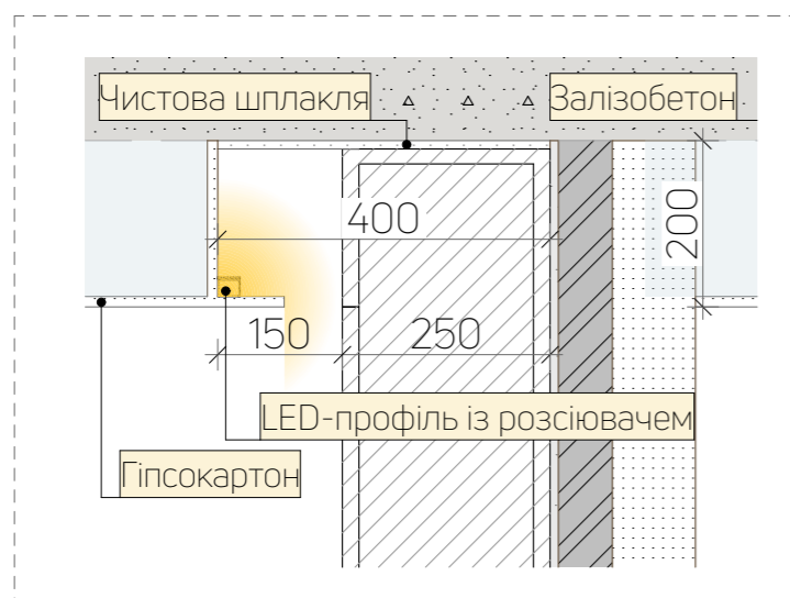
РОЗРІЗ 5-5
